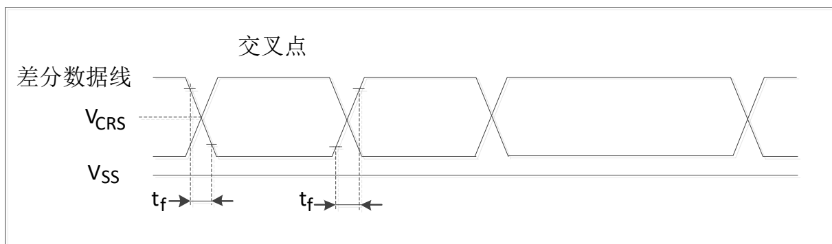
图15 USB D 时序：数据信号上升和下降的时间定义
