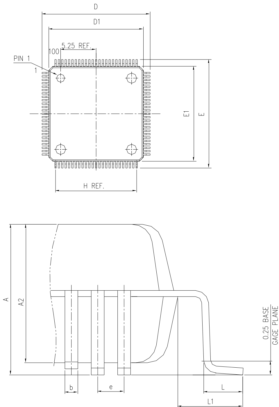
图20 LQFP100 封装图
