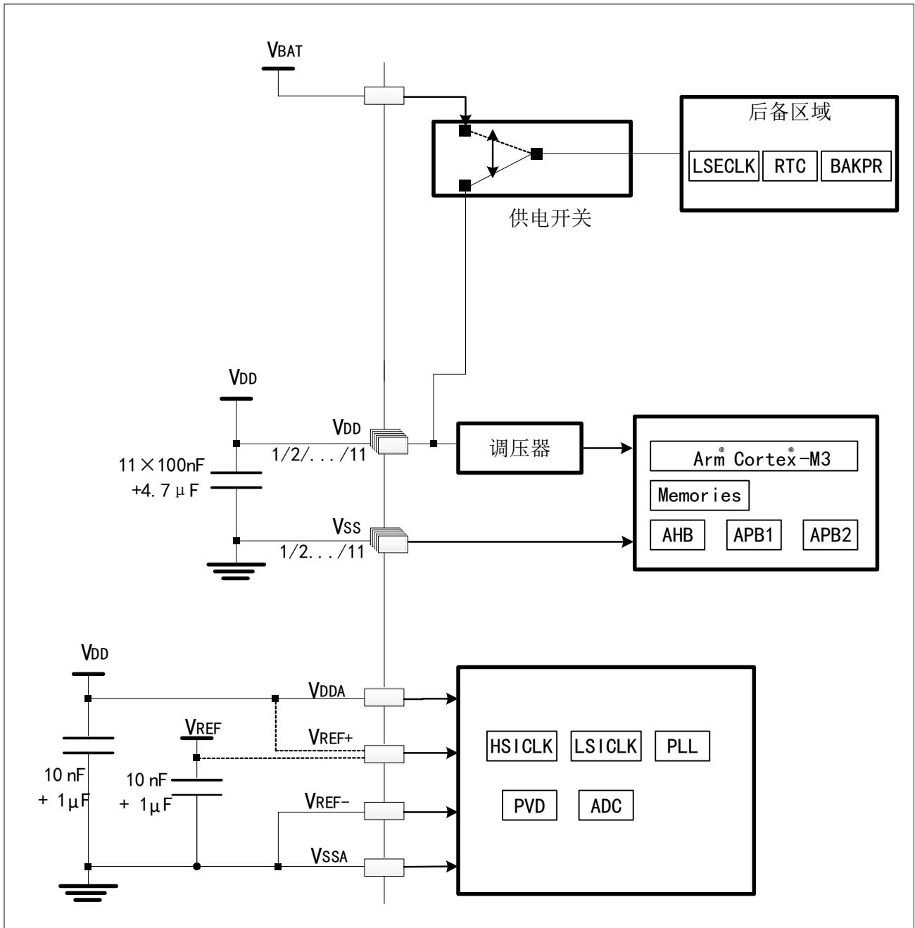
图9 供电方案
