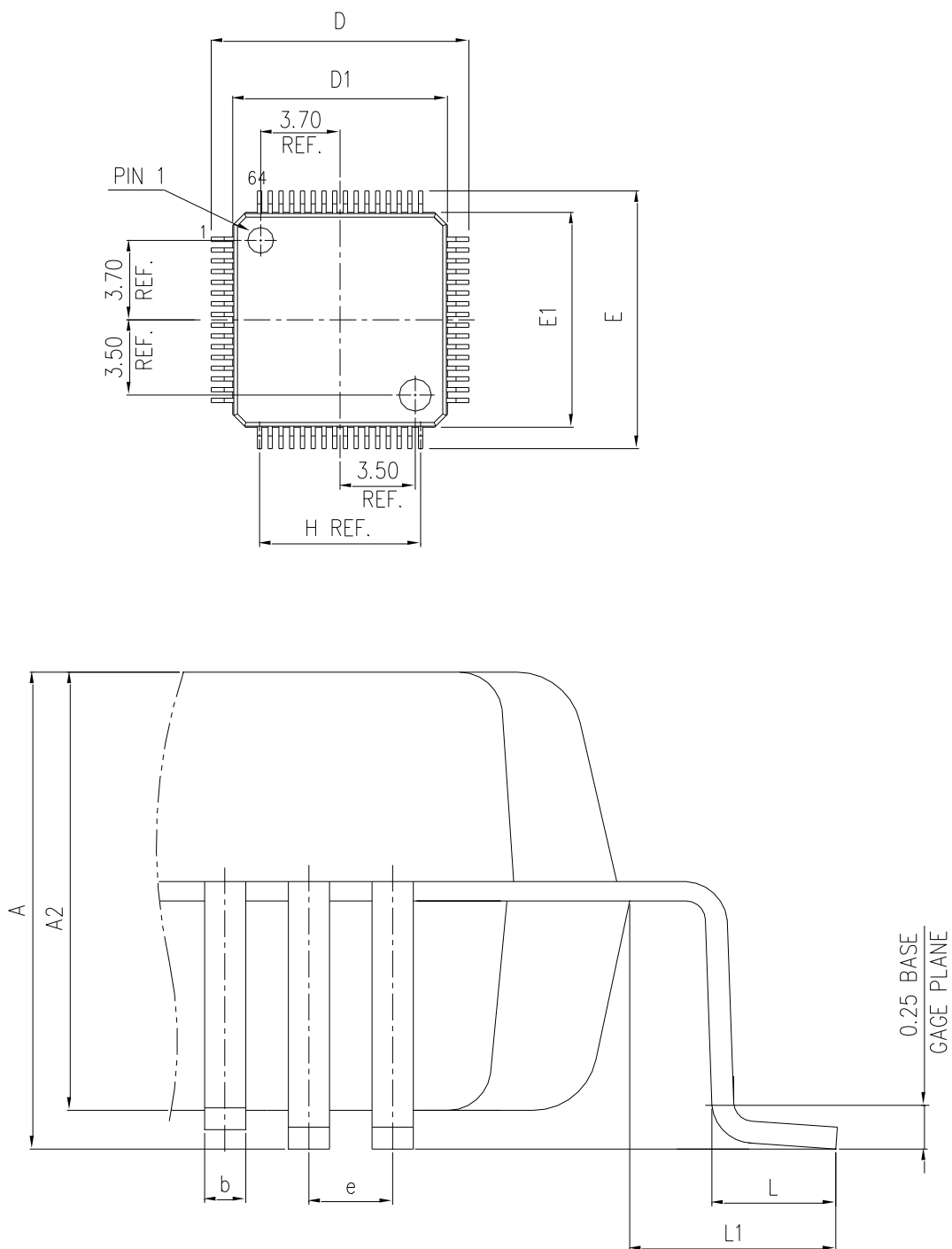
图23 LQFP64 封装图
